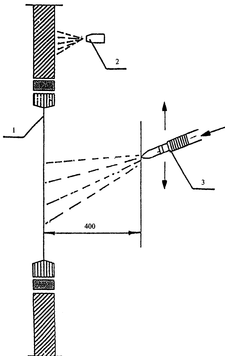
1 — образец; 2 — форсунка верхнего неподвижного ряда; 3 — подвижная форсунка
